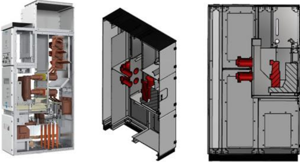
CELDAS DE SECCIONAMIENTO Y DERIVACION
